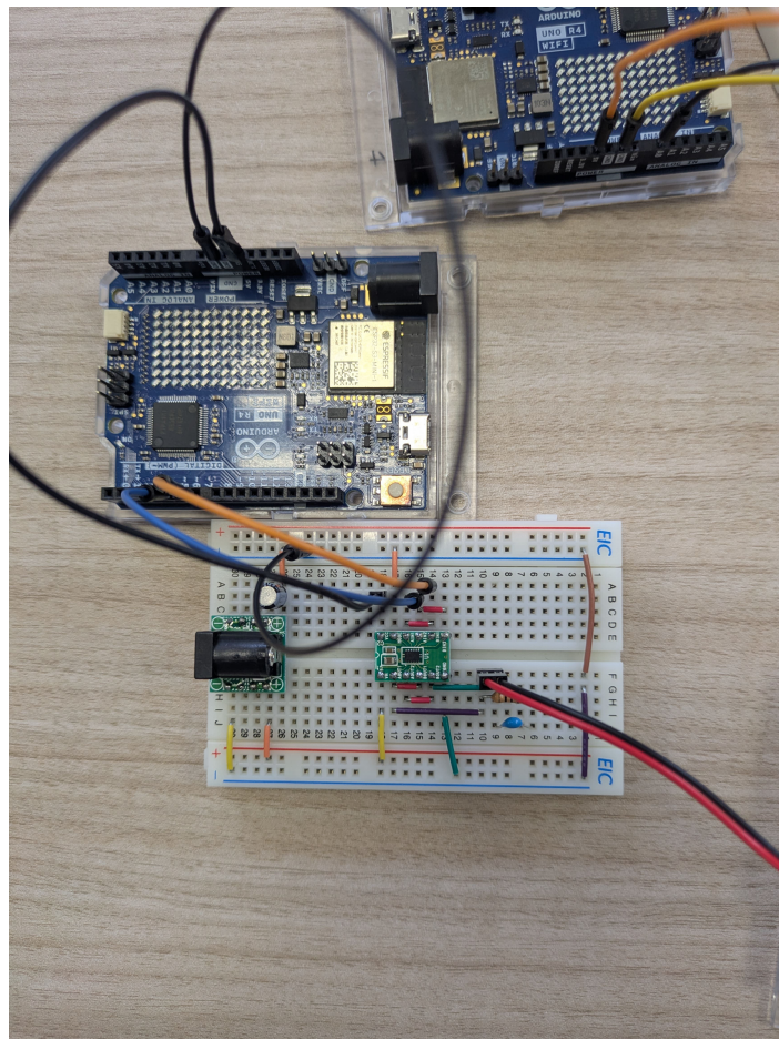
図 32 モータドライバ周辺の回路実装
