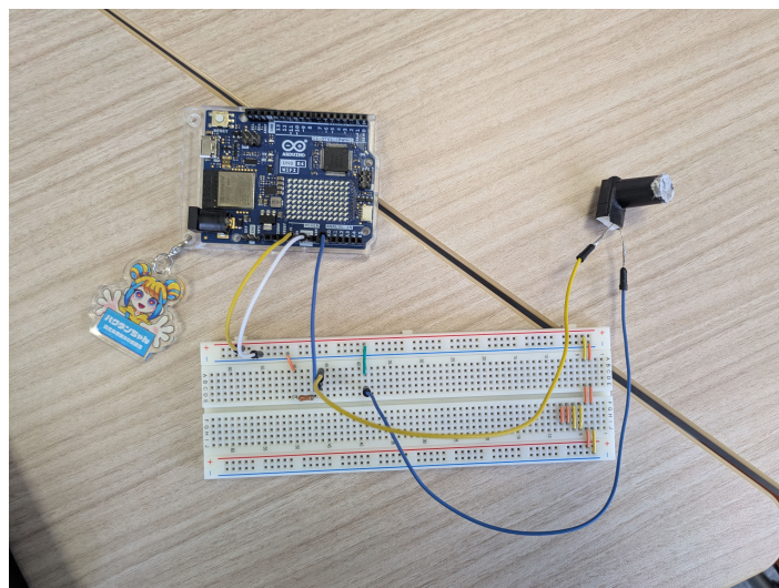
図 37 受光素子部の実装（タピオカ用の黒いストローで CdS セルを覆い、先端をティッシュペーパーで覆っている）
