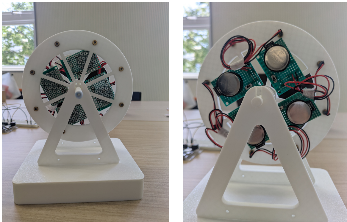
図 35 回転リングへの電池基板の実装（左：正面，右：背面．4 枚の電池基板を中心軸を囲うように十字状の対称配置とし，ボタン電池 CR2477・ホルダー・スライドスイッチを搭載している）
