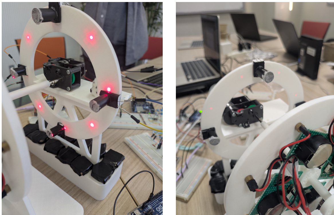
図 46 電池の消耗に伴うレーザー光量の変化（左：スイッチ ON 直後、右：時間経過後、受光部に投影された輝点の明るさが低下している）
